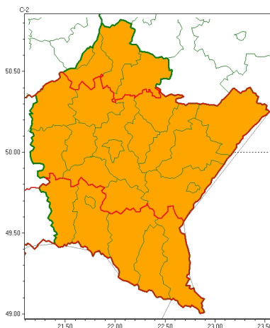
Opady marznące 2025-01-14 22:25
